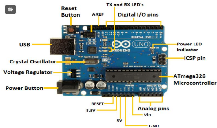
Figure 13: Arduino Uno.
