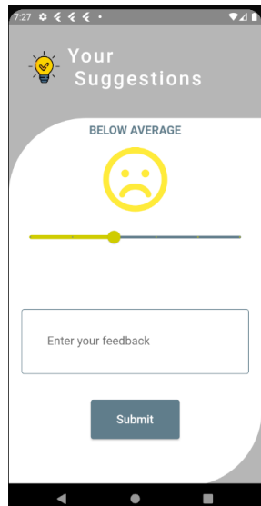
parent feedback
