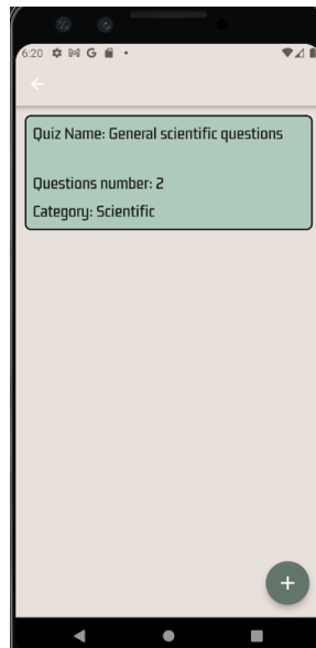
Create Quiz
