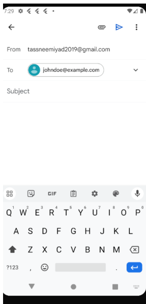
Gmail
