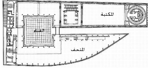
الشكل(5:6): المسقط الأفقي للدور الرابع ويحتوي على المكتبة والمتحف (المصدر: www.greatbuildings.com )
